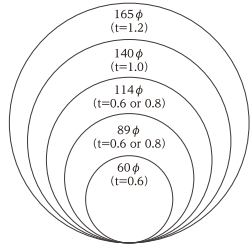
タフステン断面寸法図
