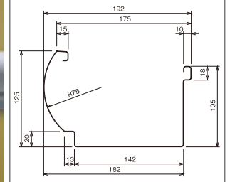
タフゾウ断面寸法
