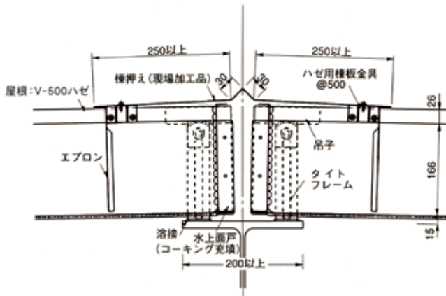
棟納め(タイトフレーム使用の場合)
