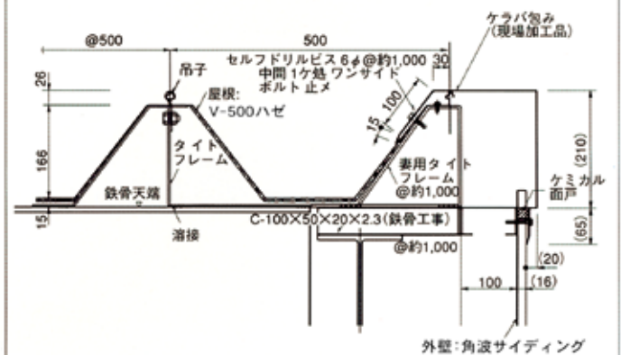
ケラバ納め
